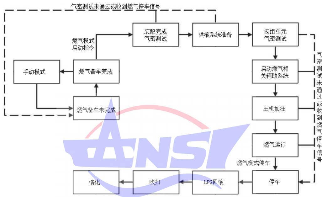
图 1 燃气切换流程框图
